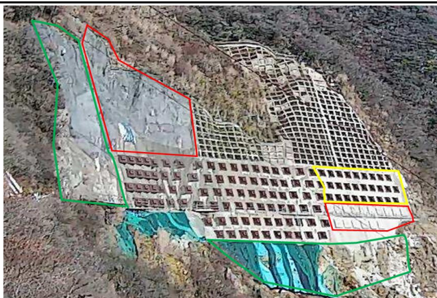
早雲山 地すべり対策工事 進捗状況
