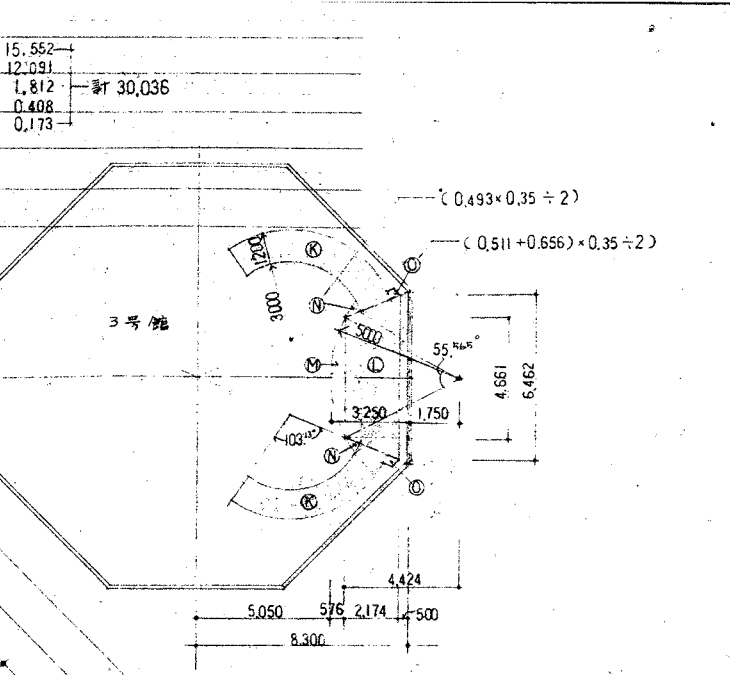
2階建物寸法図 S=1/150
